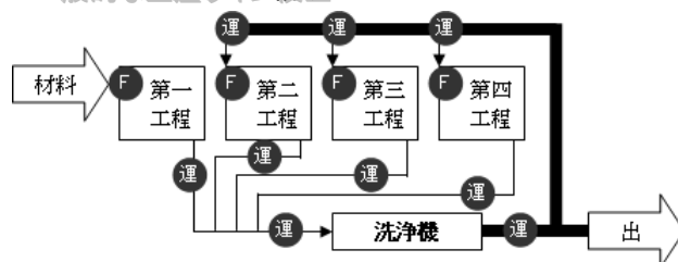
新商品使用 生産ライン構成例
