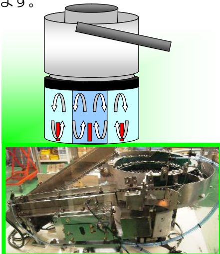
一般的な生産ライン構成
